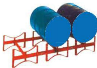
FIE 169 Drum stand Cap:1050 kgs
